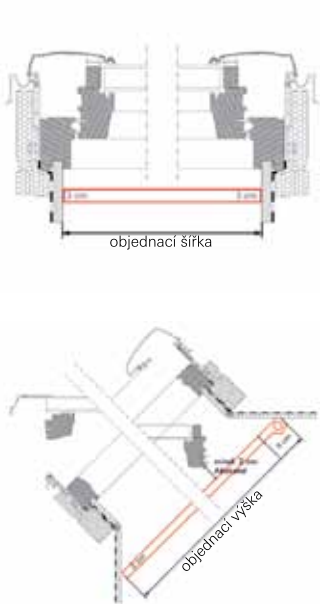
Varianta „L“ – do ostění
