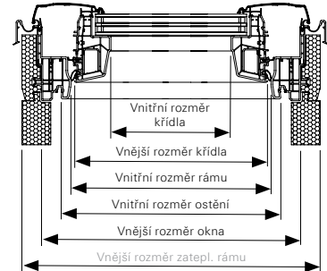
řez B-B
