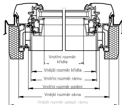
řez B-B
