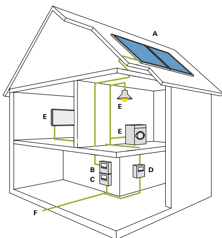
Photovoltaik-System im Überblick
